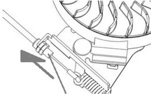
Réglage du câble du Levier de frein moteur
